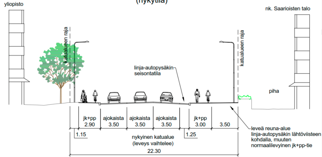
poikkileikkaus A-A (nykytila)
