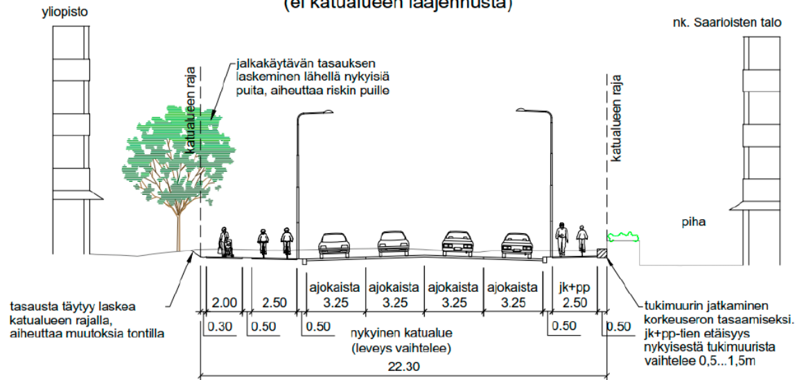
poikkileikkaus A-A (ei katualueen laajennusta)
